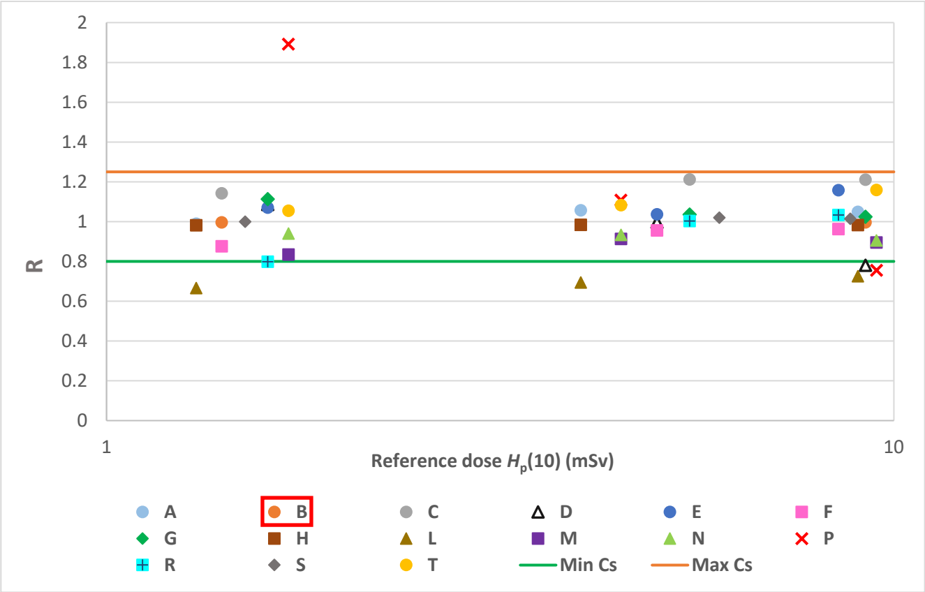
Figura 2: Curva a trombetta per i tre irraggiamenti eseguiti a qualità nota S-Cs, suddivisi in set dosimetrici, per la grandezza H_p(10) (nel riquadro rosso è indicato il set relativo all'attestato)
