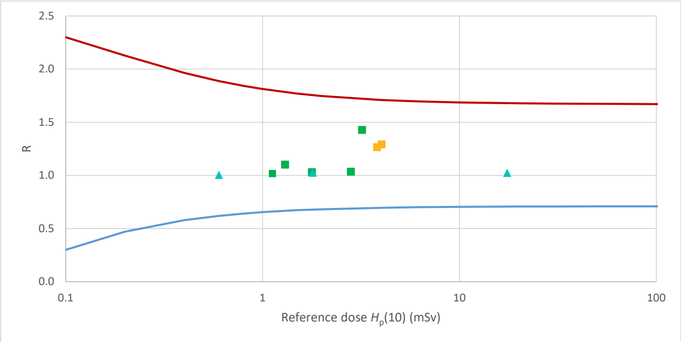
Figura 4: Curva a trombeta per i dati del set relativo all’attestato, per la grandezza H_p(10) , per gli irraggiamenti a qualità nota (qualità di riferimento S-Cs).
