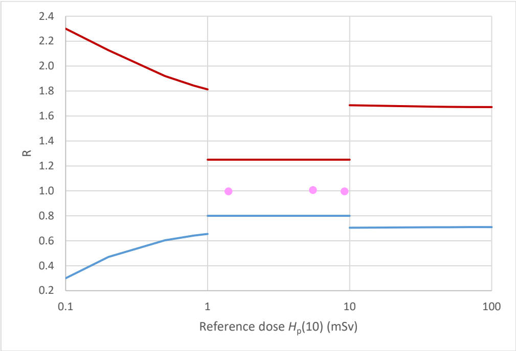
Figura 4: Curva a trombeta per i dati del set relativo all’attestato, per la grandezza H_p(10) , per gli irraggiamenti a qualità nota (qualità di riferimento S-Cs).
